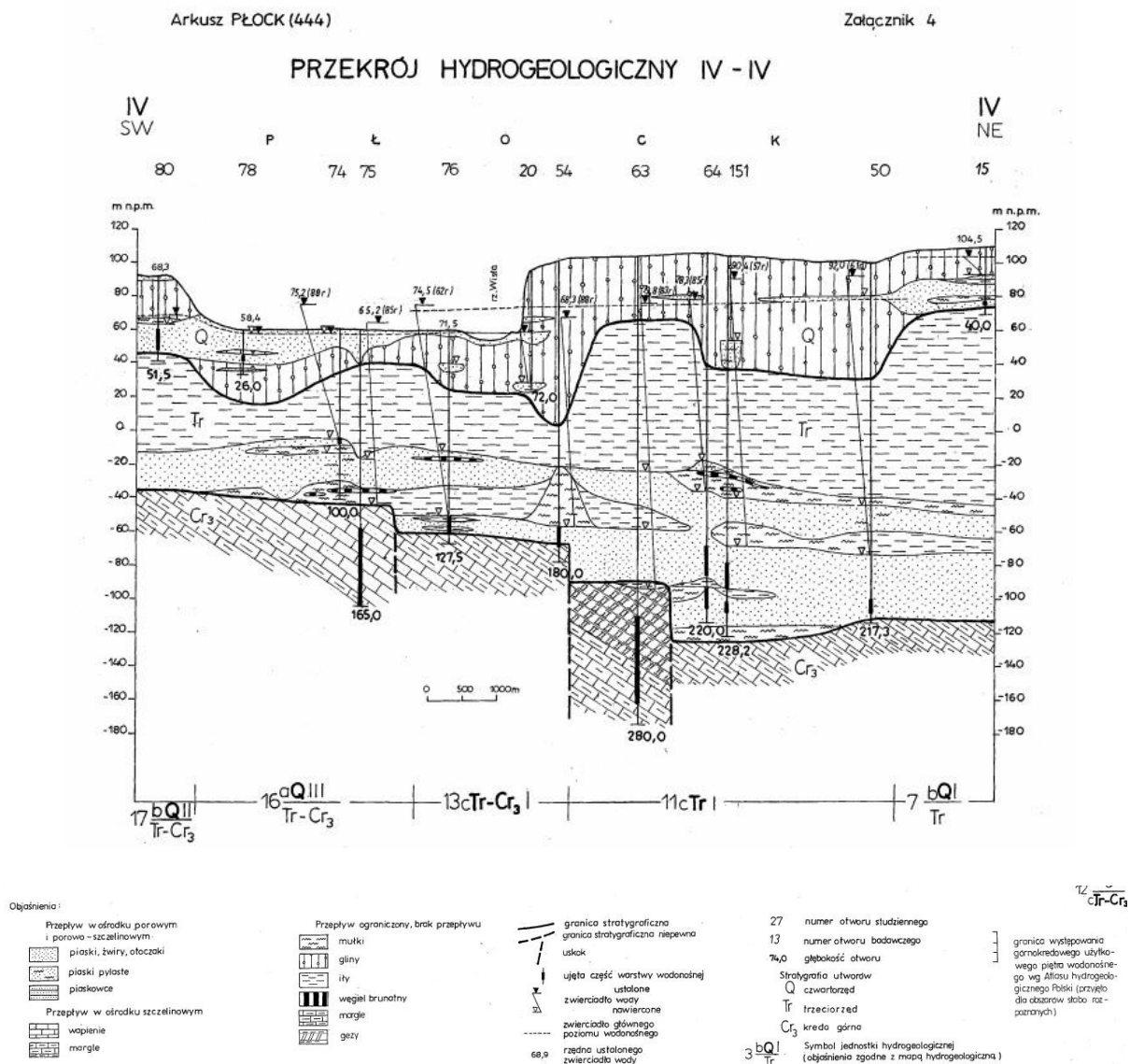
Ryc. 1. Przekrój geologiczny.
