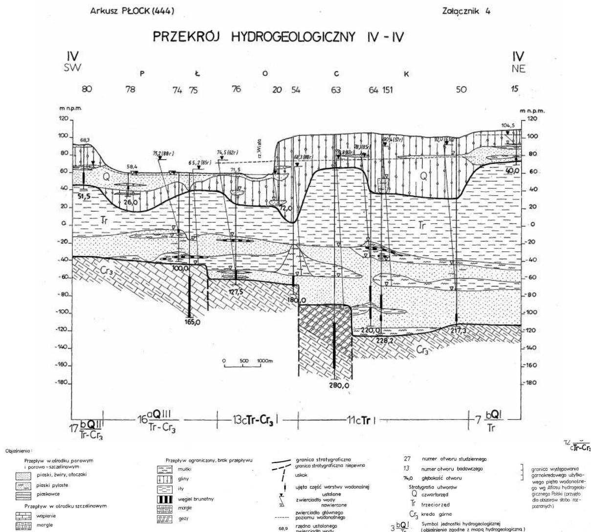
Ryc. 1. Przekrój geologiczny.
