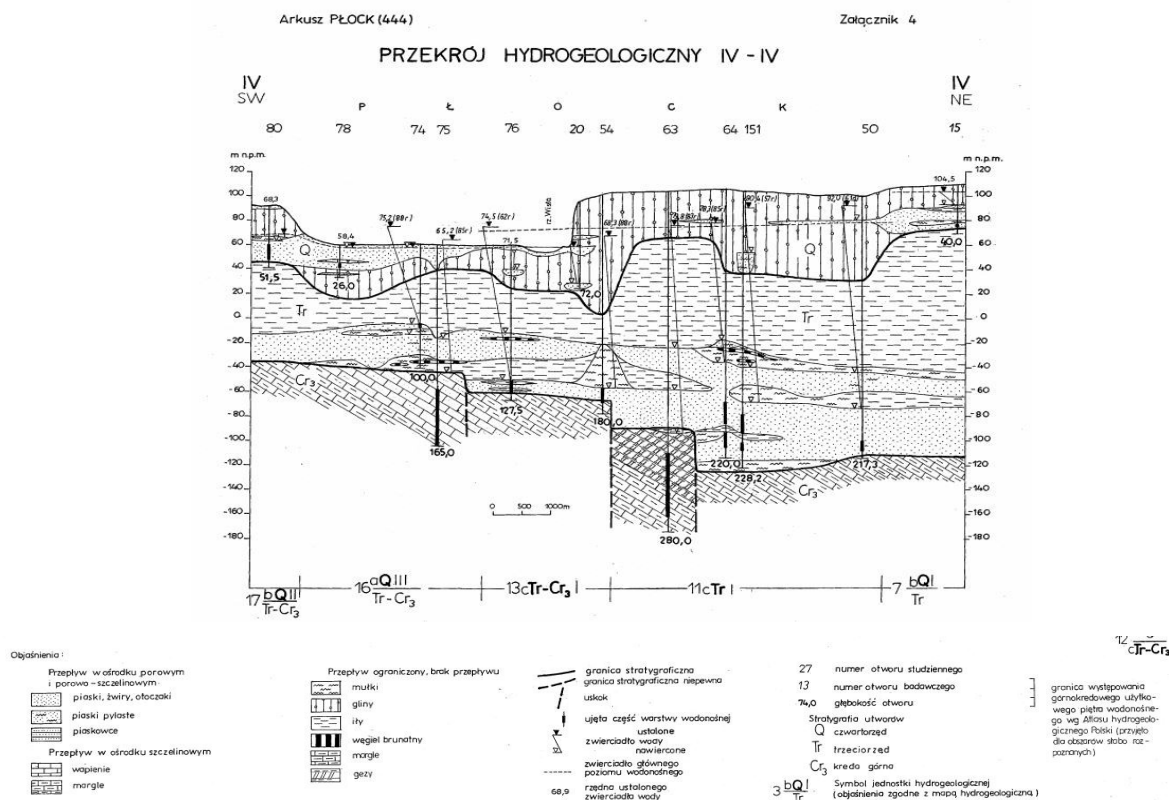
Ryc. 1. Przekrój geologiczny.
