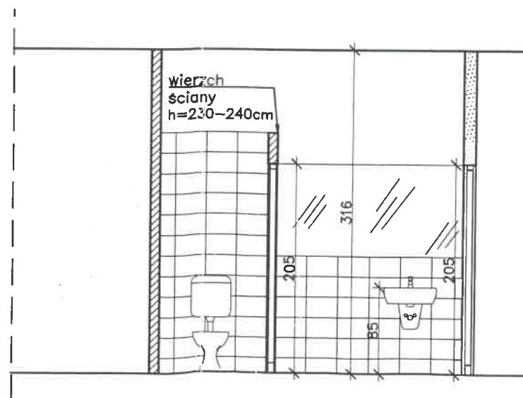
Przekrój a - a
